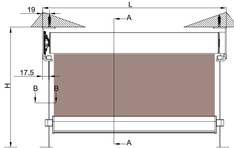
supporto a parete - wall bracket
