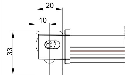
pedino a pavimento - floor bracket B-B
